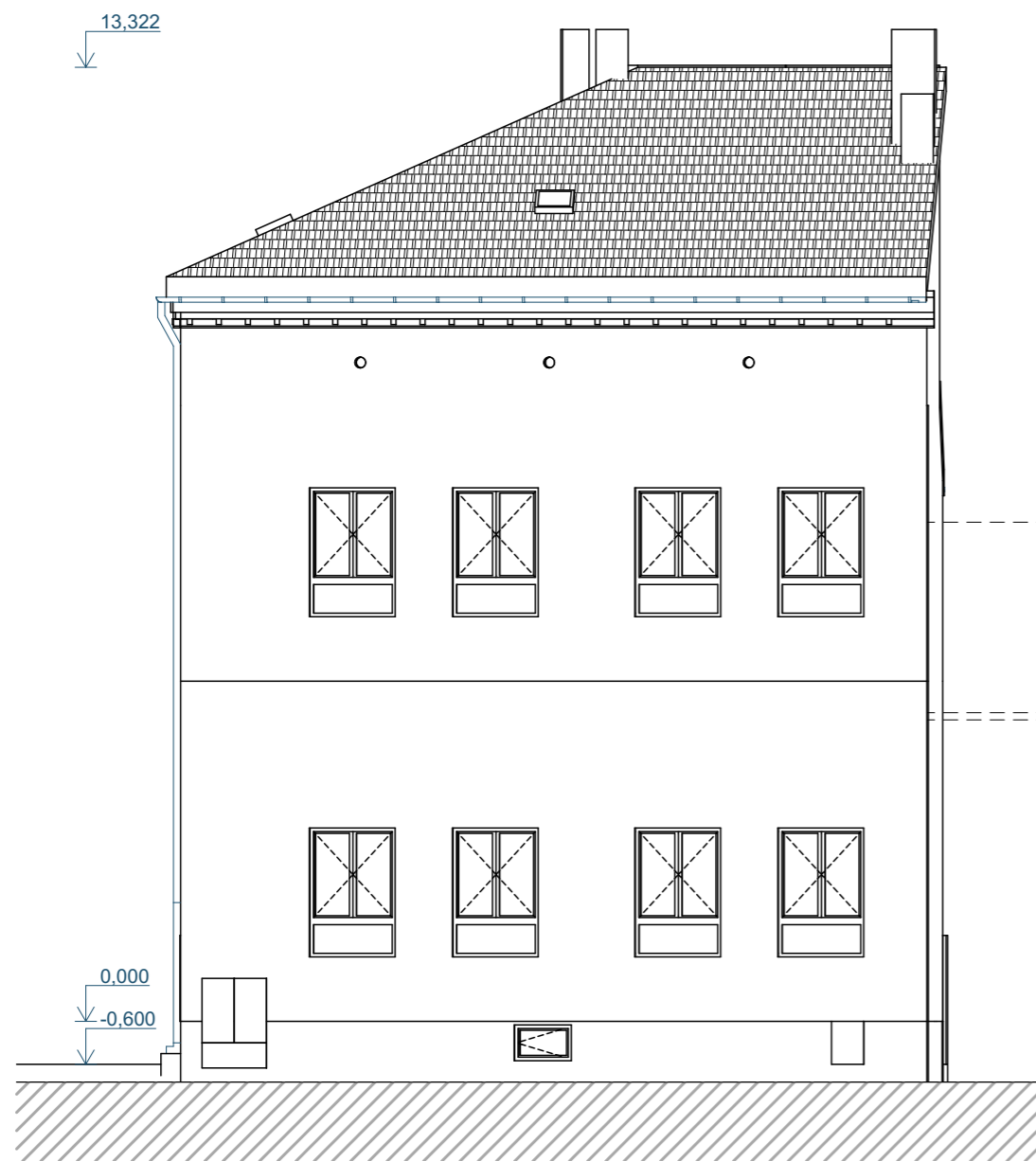
POHLED SEVEROVÝCHODNÍ - STÁVAJÍCÍ STAV.
