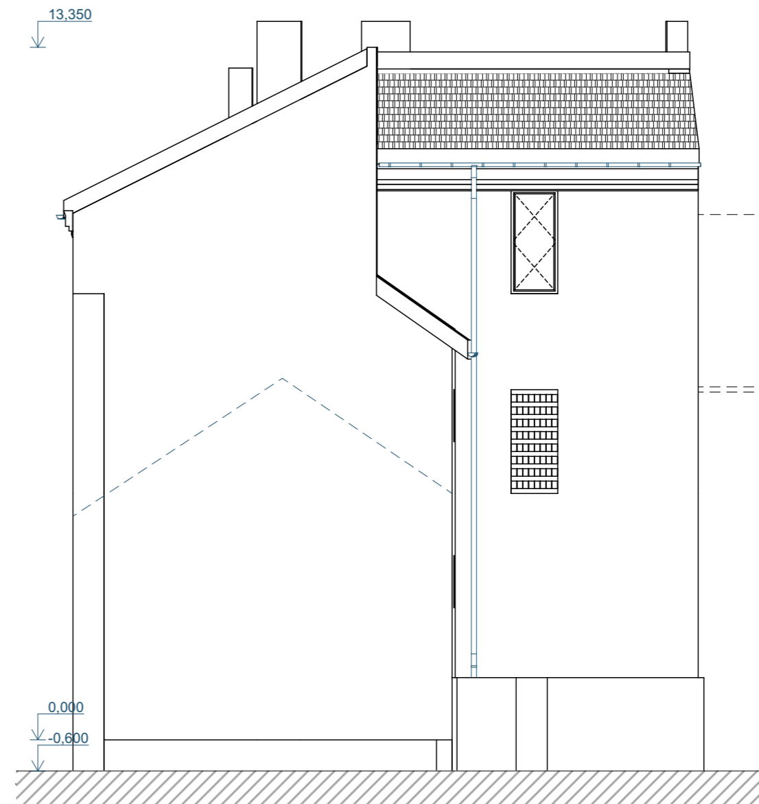
POHLED SEVEROZÁPADNÍ - STÁVAJÍCÍ STAV.
